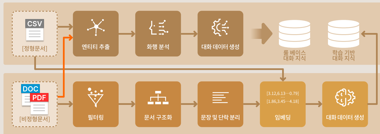
대화데이터 생성 도구
